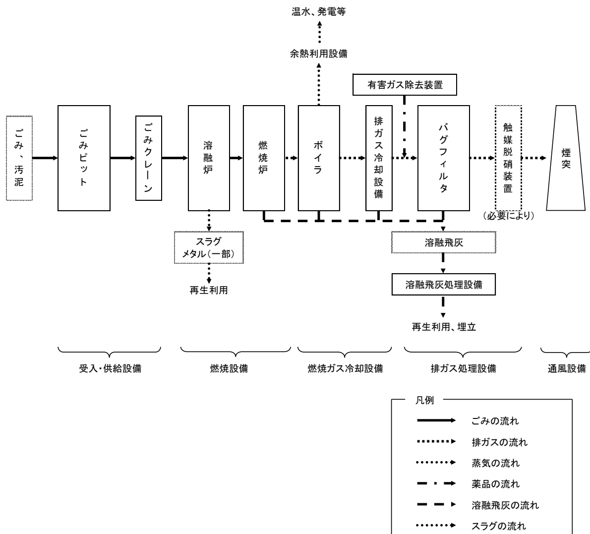
図 5-10 ガス化溶融施設（シャフト炉式）の処理フロー（例）
