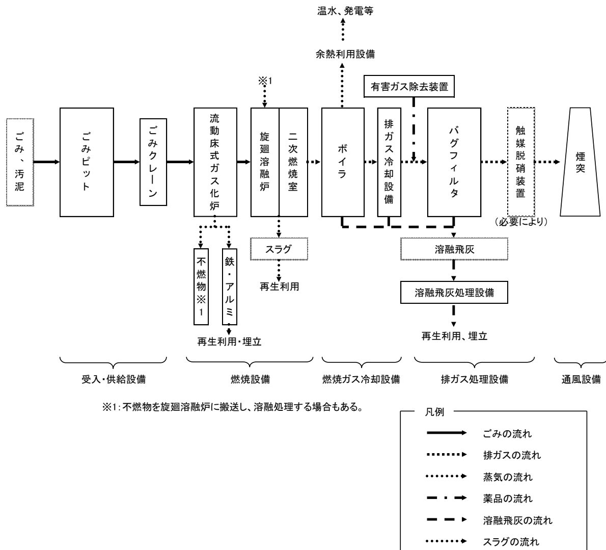
図5-11 ガス化溶融施設（流動床式）の処理フロー（例）
