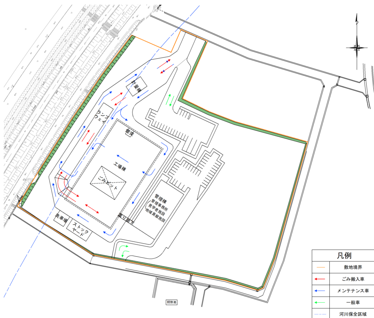
図 6-1 配置計画図 (S=1/2000)
